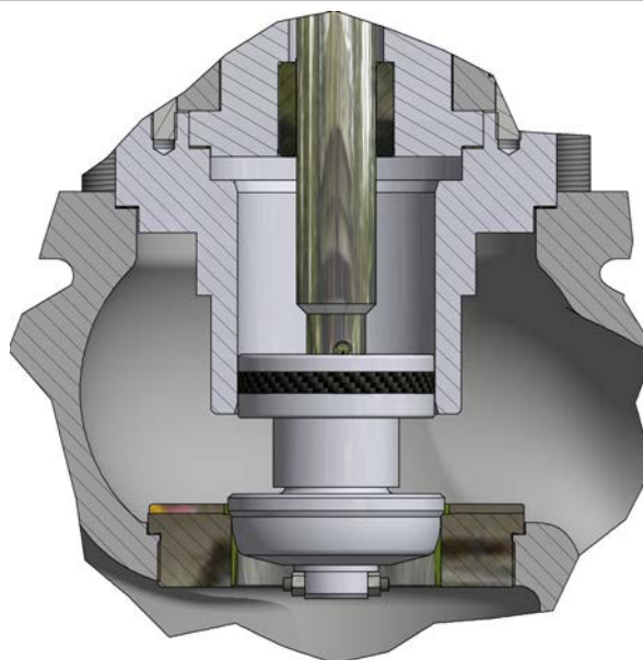
Otturatore bilanciato
